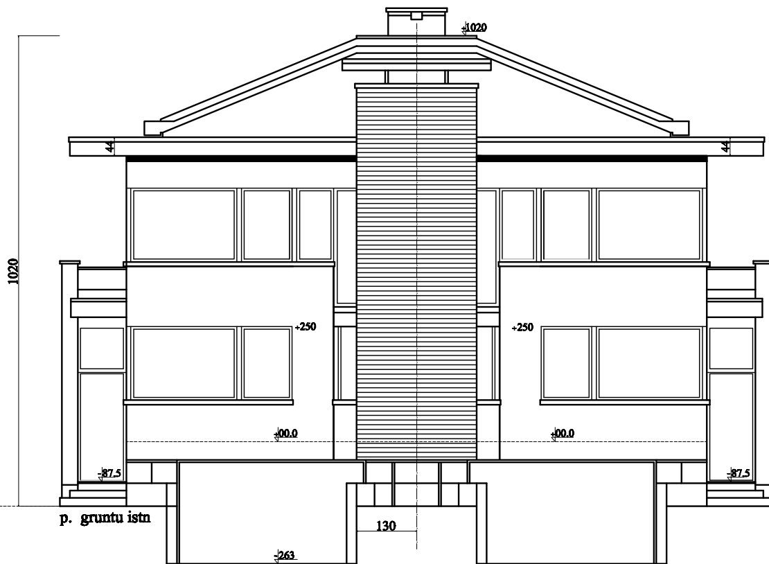
SEG. L ELEVACJA OD STRONY WJAZDU SEG. P SKALA 1:100
